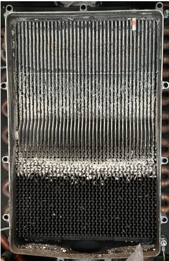
VOOR — Aluminiumoxide-ophoping
